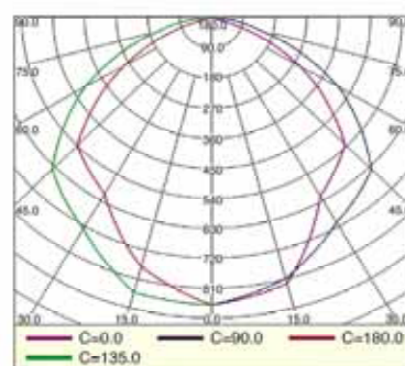
SLI-25W/765配光曲線
