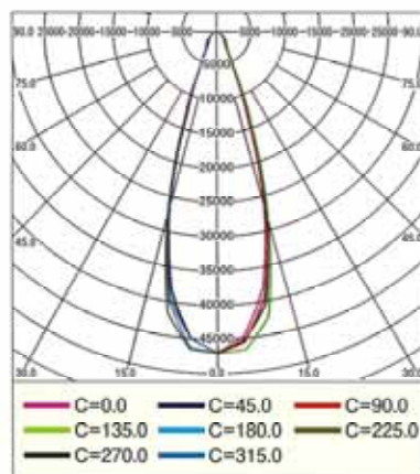
FLI-250W/765配光曲線 (40°レンズ適用の場合)
